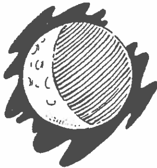
la Lune 11.
