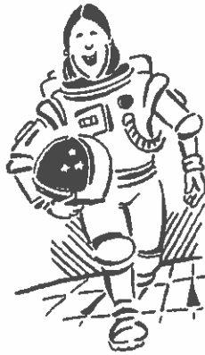
une astronaute 2.
