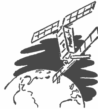
un satellite 3.
