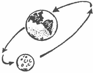
une orbite 10.
